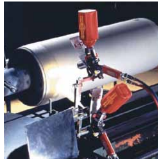
Газотермическое напыление Eutalloy RW с помощью аппарата CDS 8000
