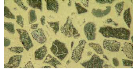
Микроструктура сплава с карбидами вольфрама
